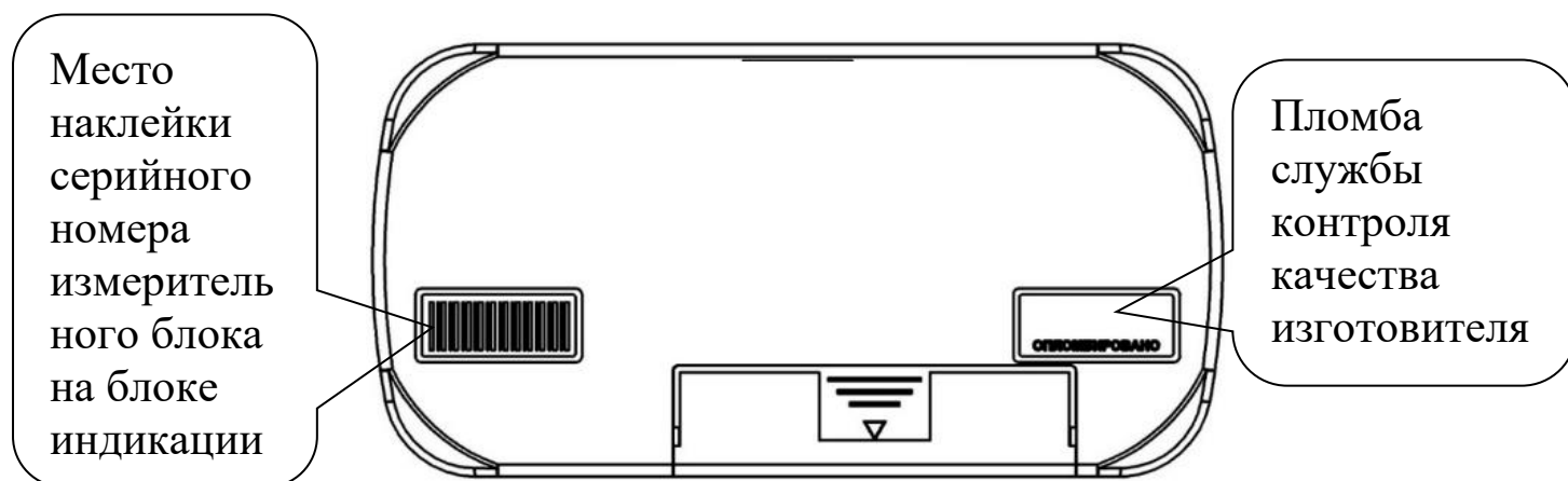
Рисунок 4 - Пломбировка блока индикации Милур Т и место наклейки серийного номера измерительного блока, к которому прикреплен блок индикации
