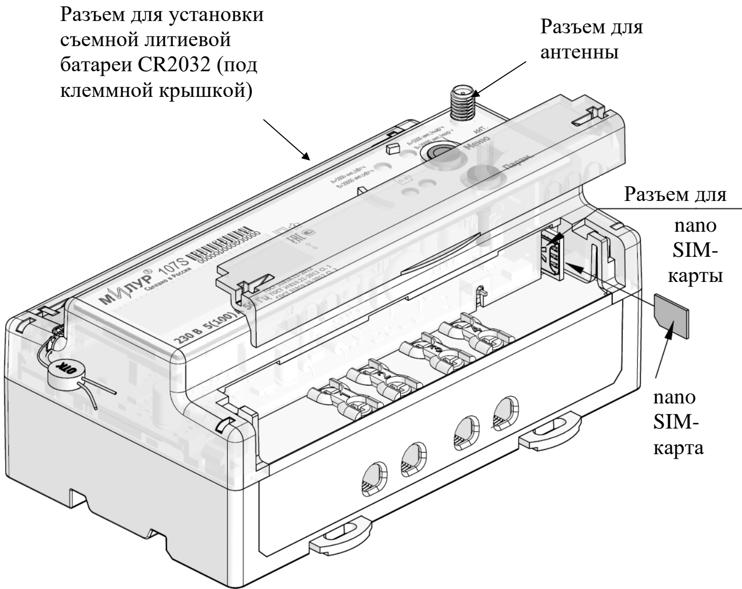
Рисунок 17 - Счетчик в корпусе 9mTH35
