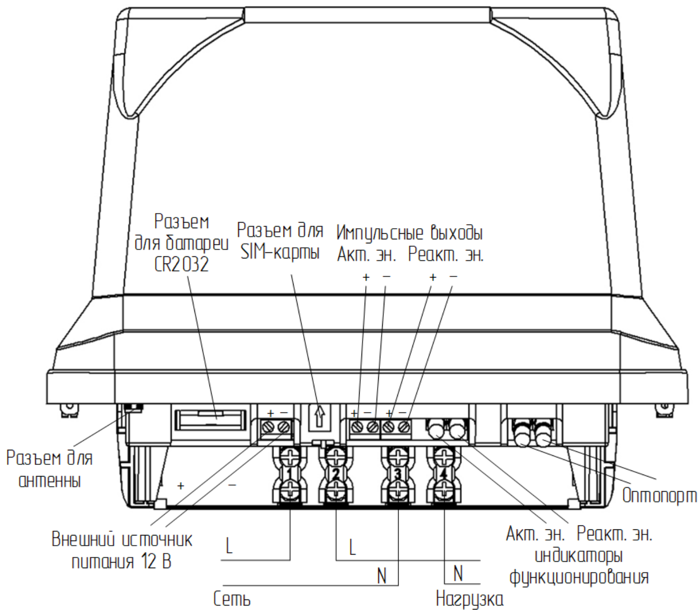
Рисунок 8 - Общий вид, назначение клемм и схема подключения к сети счетчика в корпусе SPLIT
