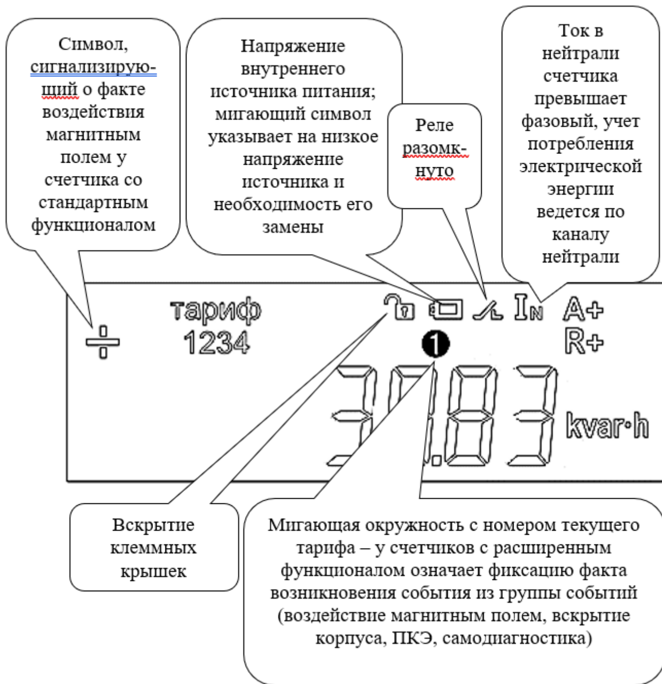
Рисунок 11 - Пример отображения символов событий для счетчика внутренней установки в корпусе 7мТН35, 9мТН35
